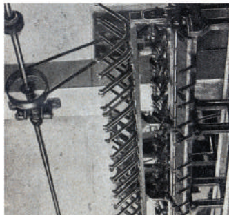
Шпулярная машина (собрана цепиком в «Интергильпо»)
